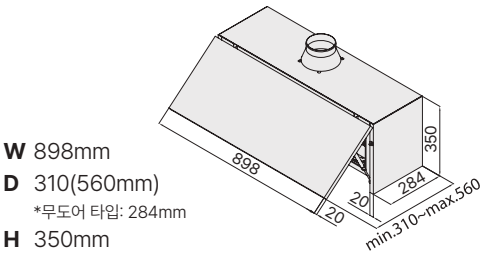
무도어 타입 HDH-90S(T1NB)
