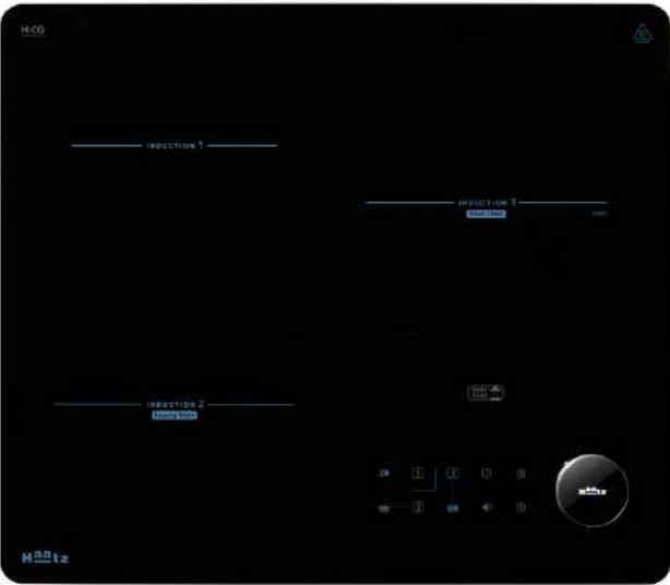
인덕션 3구(대화구 1구 1,500W(터보 2,000W), 중화구 1구 1,500W, 소화구 1구 1,100W)
