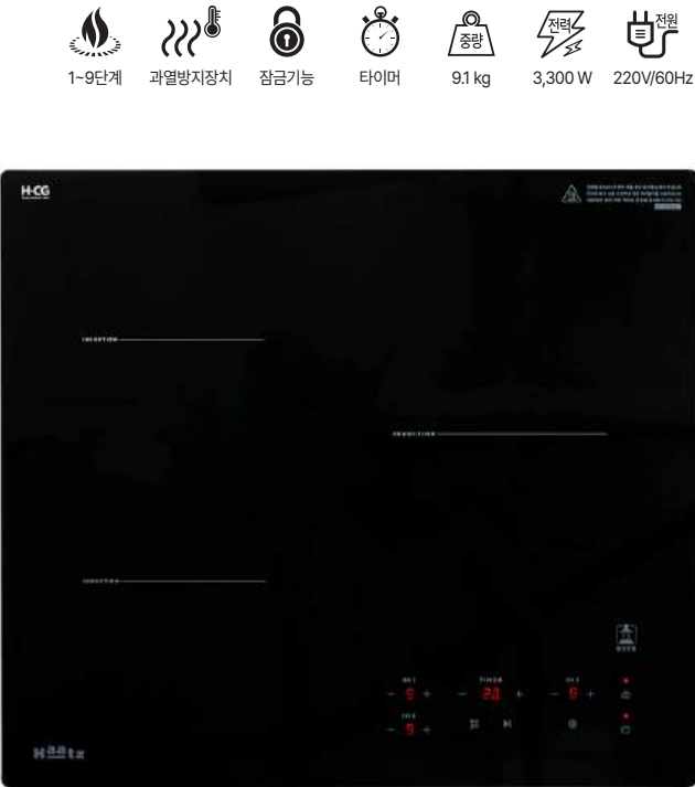
인덕션 3구(대화구 1구 1,800W(부스터 2,000W), 중화구 2구(좌상 1,500W, 좌하 1,500W))
