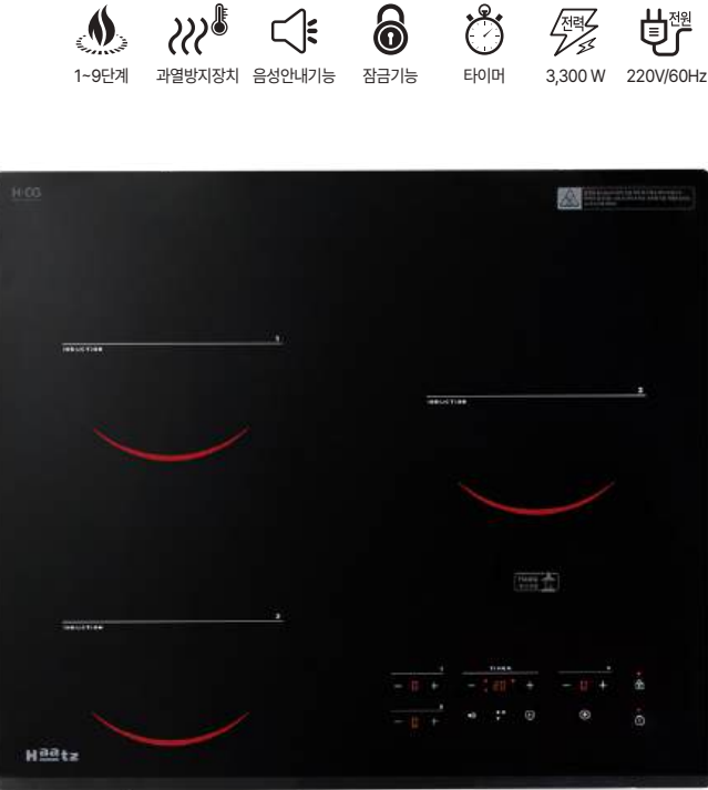
인덕션 3구(대화구 1구 1,800W(터보 2,200W), 중화구 2구(좌상 1,500W, 좌하 1,500W))
