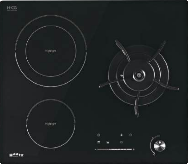
가스 1구(대버너), 하이라이트 2구(대버너 2,000W, 소버너 1,100W)
