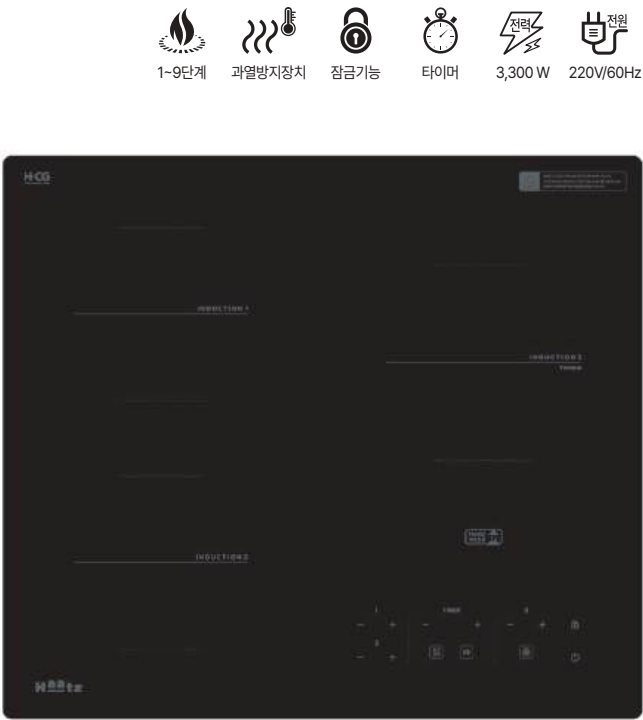
인덕션 3구(대화구 1구 1,800W(터보 2,000W), 중화구 2구(좌상 1,500W, 좌하 1,500W))
